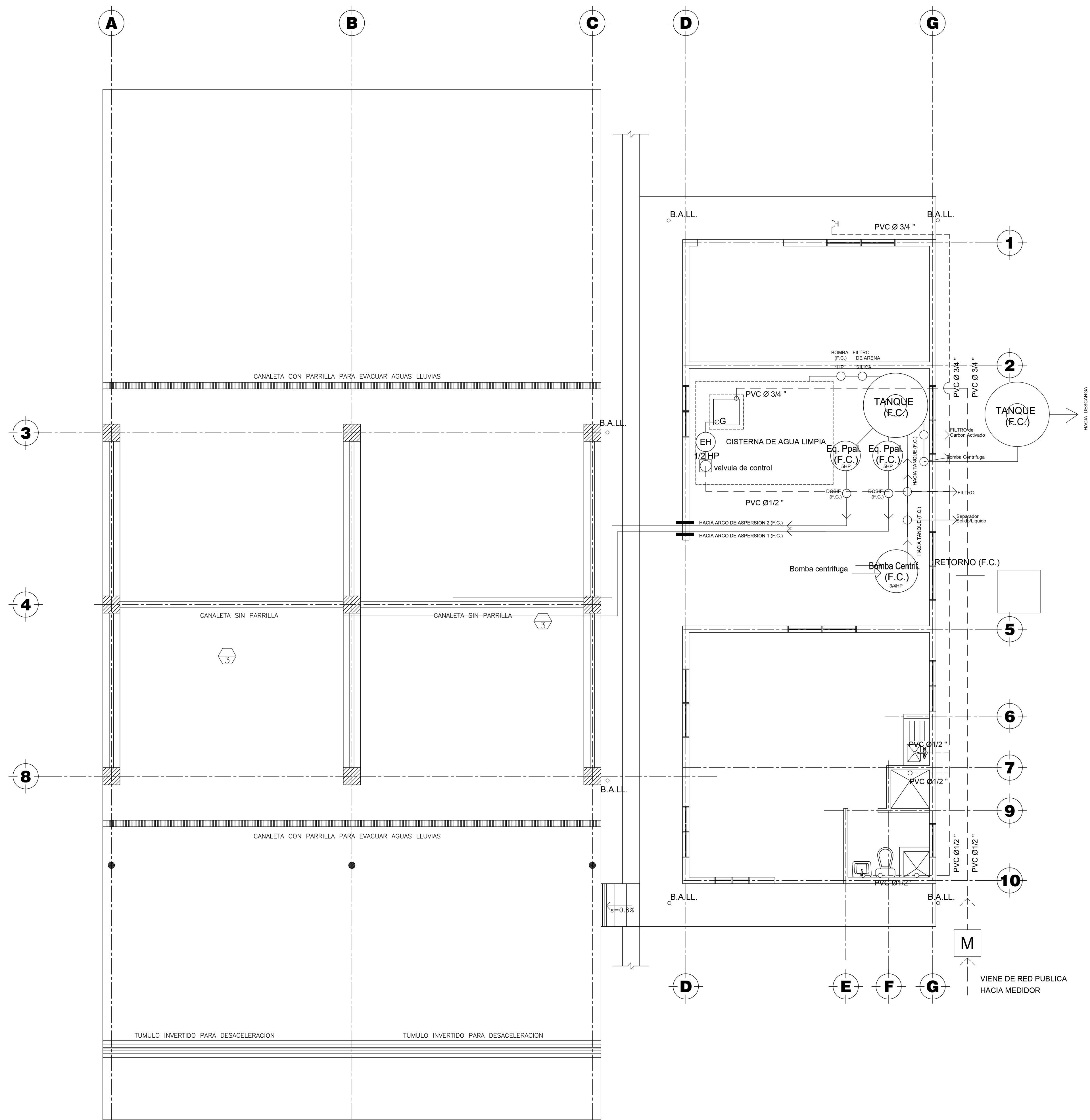
DISTRIBUCION DE AGUA POTABLE Y REINYECCION DE AGUA TRATADA ESC. 1:50
