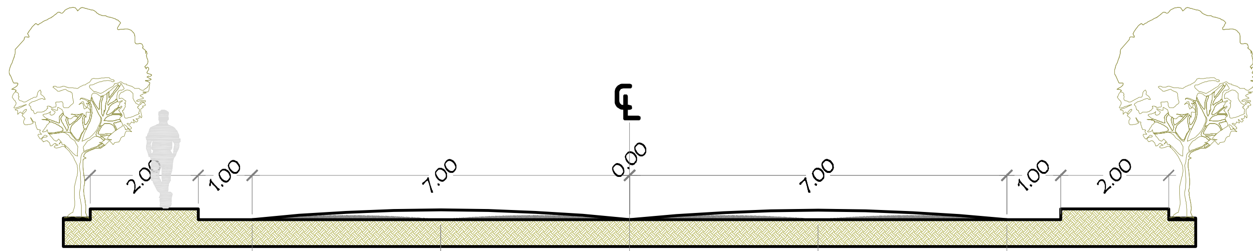
SECCIÓN VÍA PANAMERICANA
