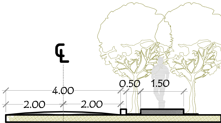
SECCIÓN VÍA MARGINAL
